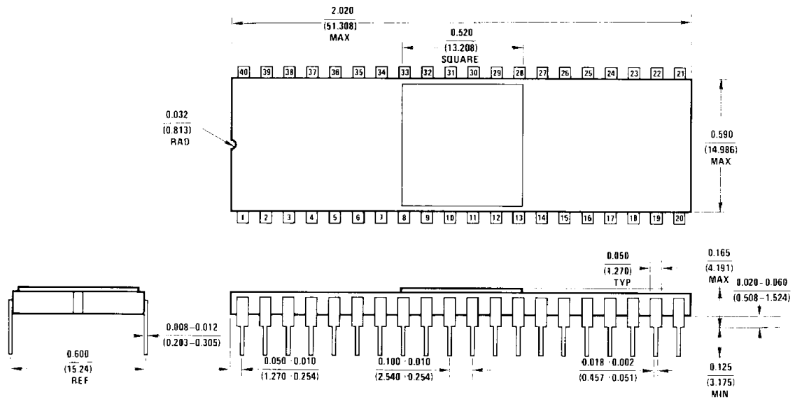
Ceramic Dual-In-Line Package (D) Order Number INS1771D-1
